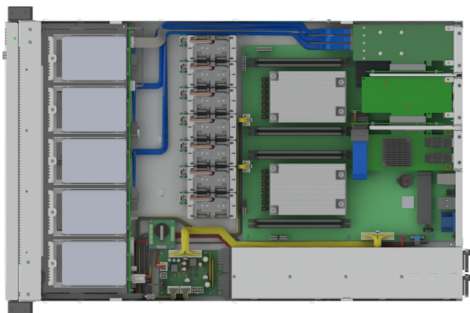
Сервер "НОРСИ-ДРАКОН" 4LFF / Вид сверху
